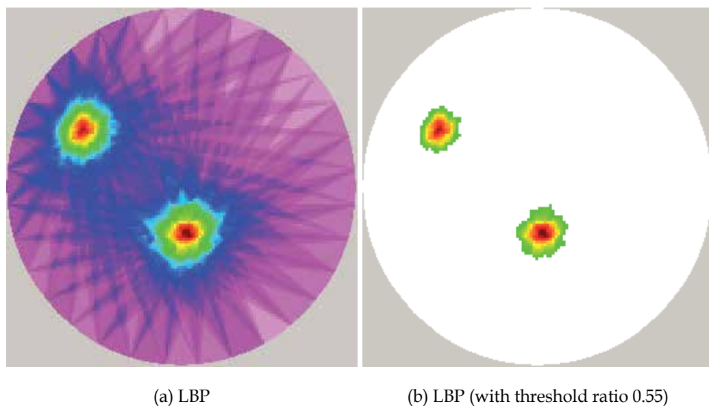
Fig. 17. Dual gas hold-up
