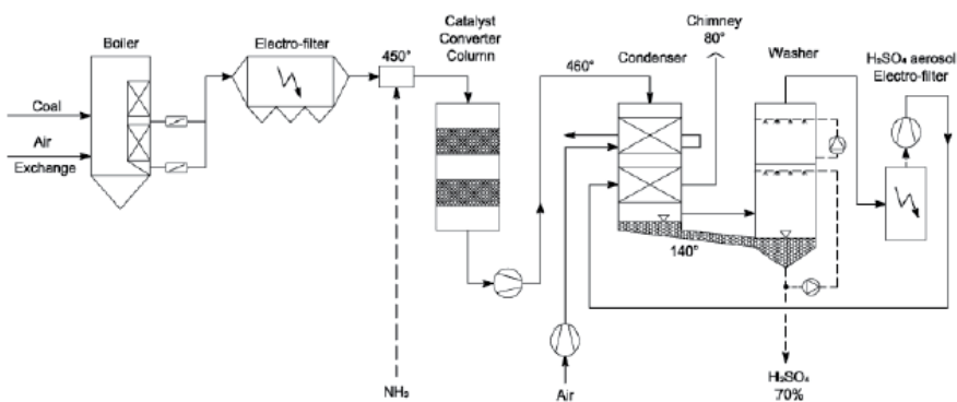
Fig. 18. DESONOX installation diagram.
