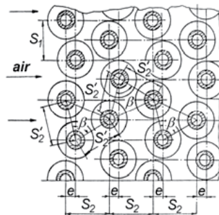
Fig. 4. Zigzag tube arrangement (Kuntysh & Kuznetsov, 1992)
