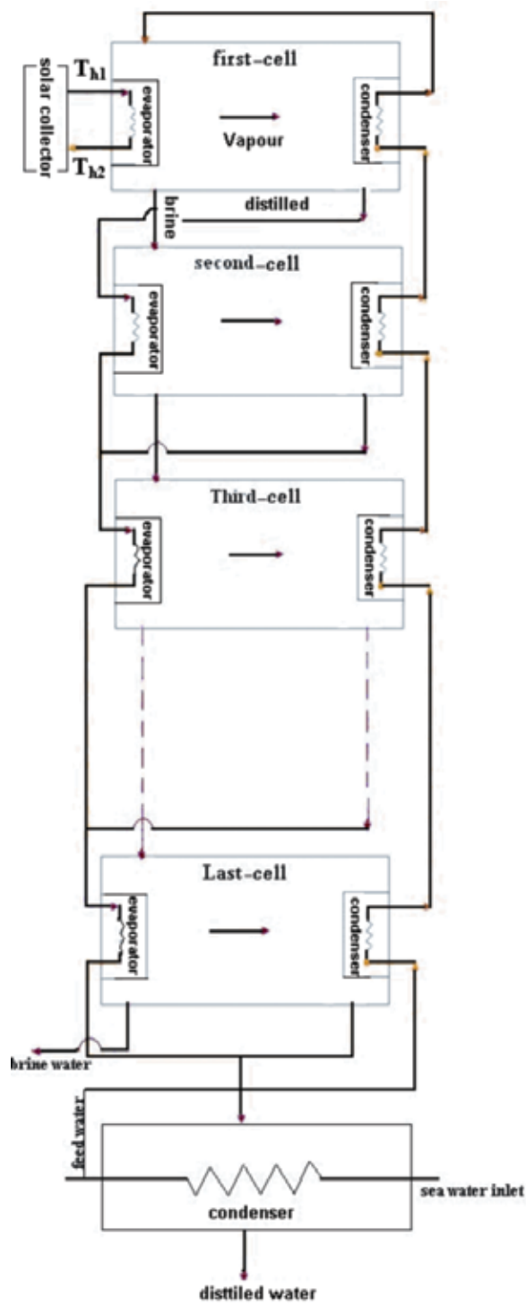
Fig. 1. Schematic diagram of MED plant
