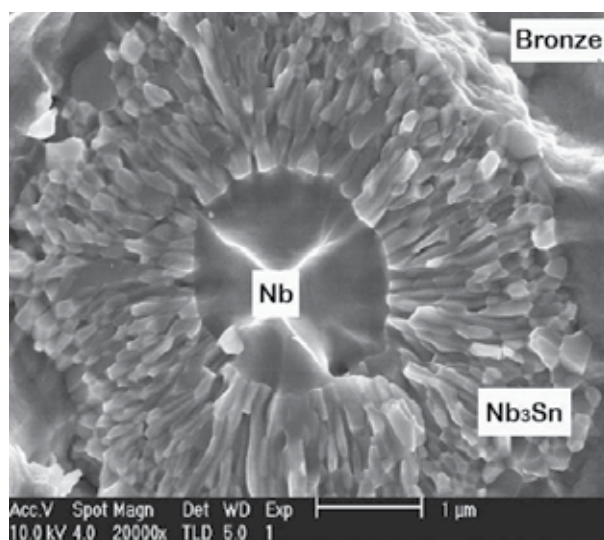
Fig. 1. Grain morphology of Nb 3 Sn layer (Flükiger et al., 2008).
