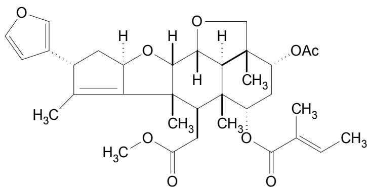
salannin
