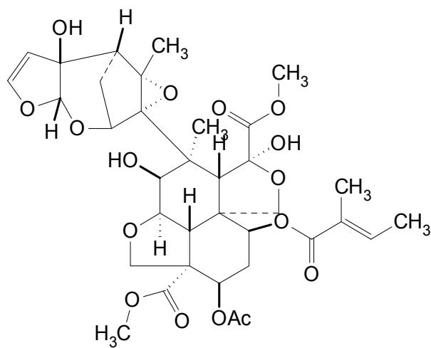
azadirachtin A
