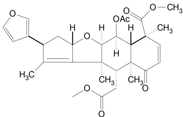
nimbin
