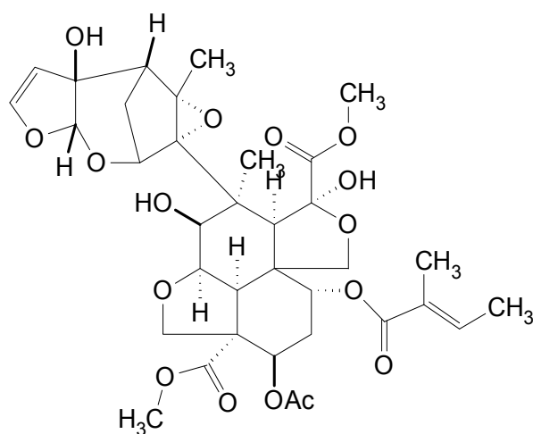
azadirachtin B
