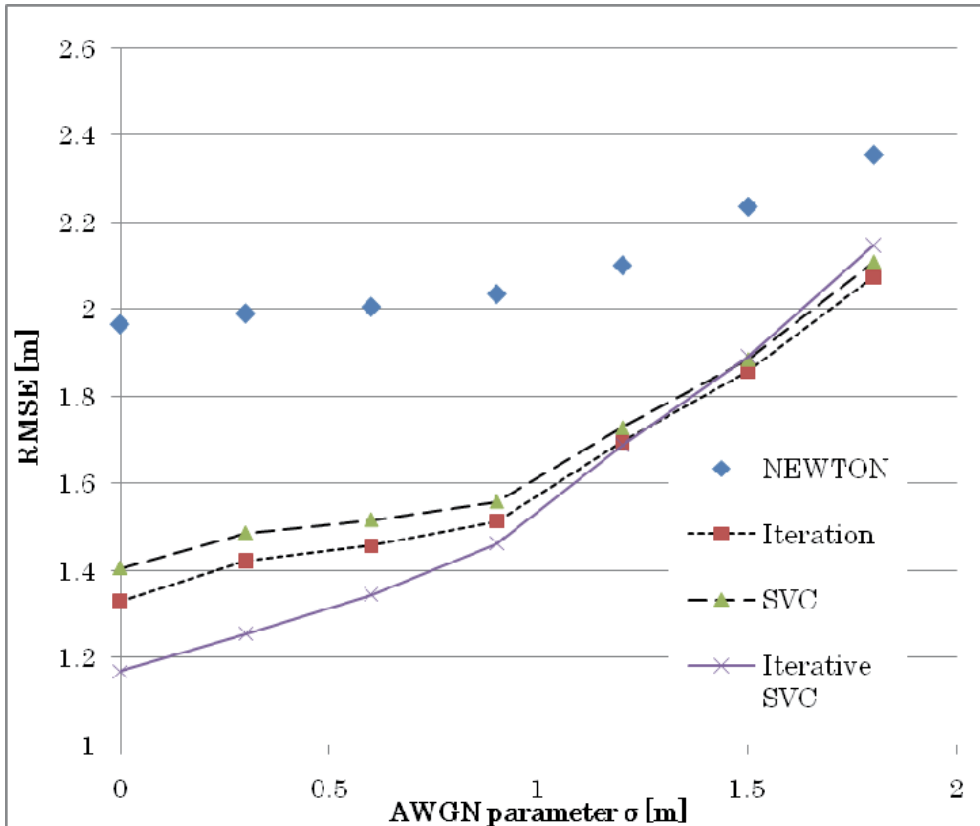
Fig. 9. RMSE evaluation changing AWGN parameter
