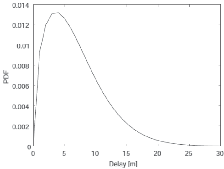
Fig. 5. IEEE.802.15.4a propagation PDF CM2(NLOS)
