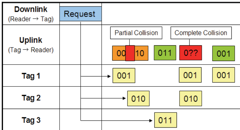
(a) (Pure) ALOHA
