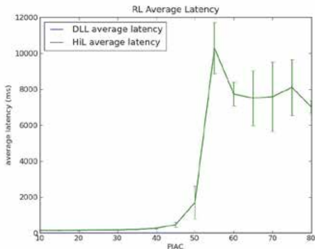
Fig. 29. RL avg. latency - scenario PIAC.
