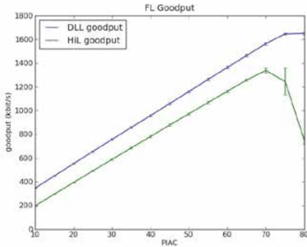
Fig. 26. FL goodput - scenario PIAC.
