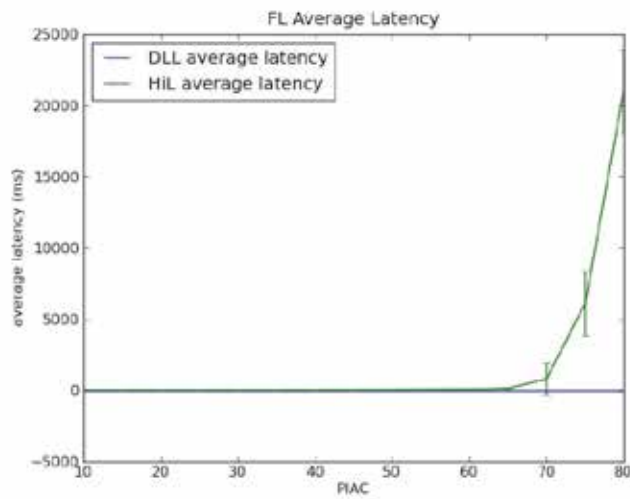
Fig. 28. FL avg. latency - scenario PIAC.
