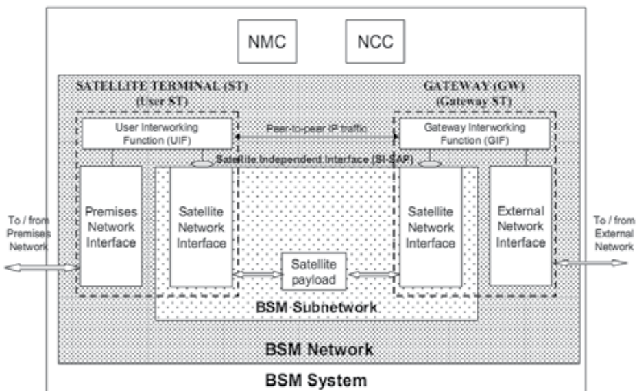
Fig. 1. BSM reference model (ETSI, 2007).
