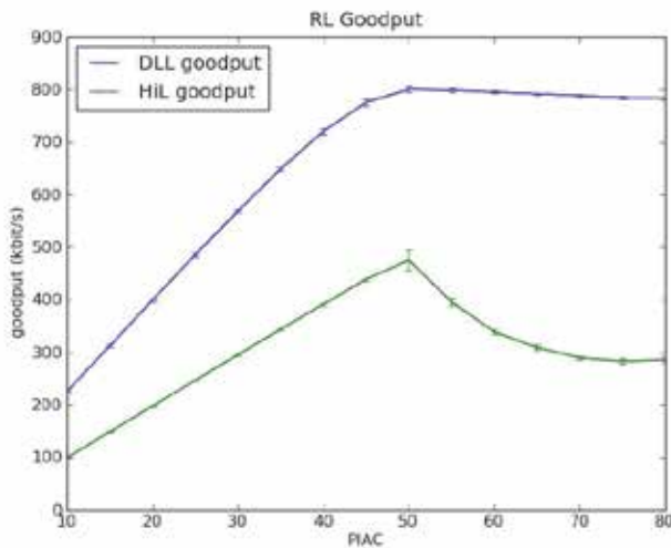
Fig. 27. RL goodput - scenario PIAC.
