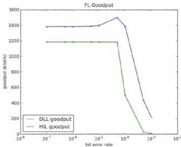
Fig. 18. FL Goodput - scenario BER.
