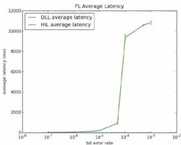
Fig. 20. FL avg. latency - scenario BER.
